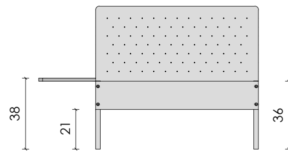
Prospetto frontale
