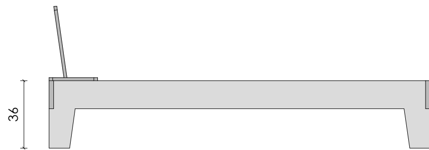
Prospetto laterale
