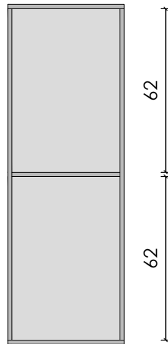
Prospetto frontale
